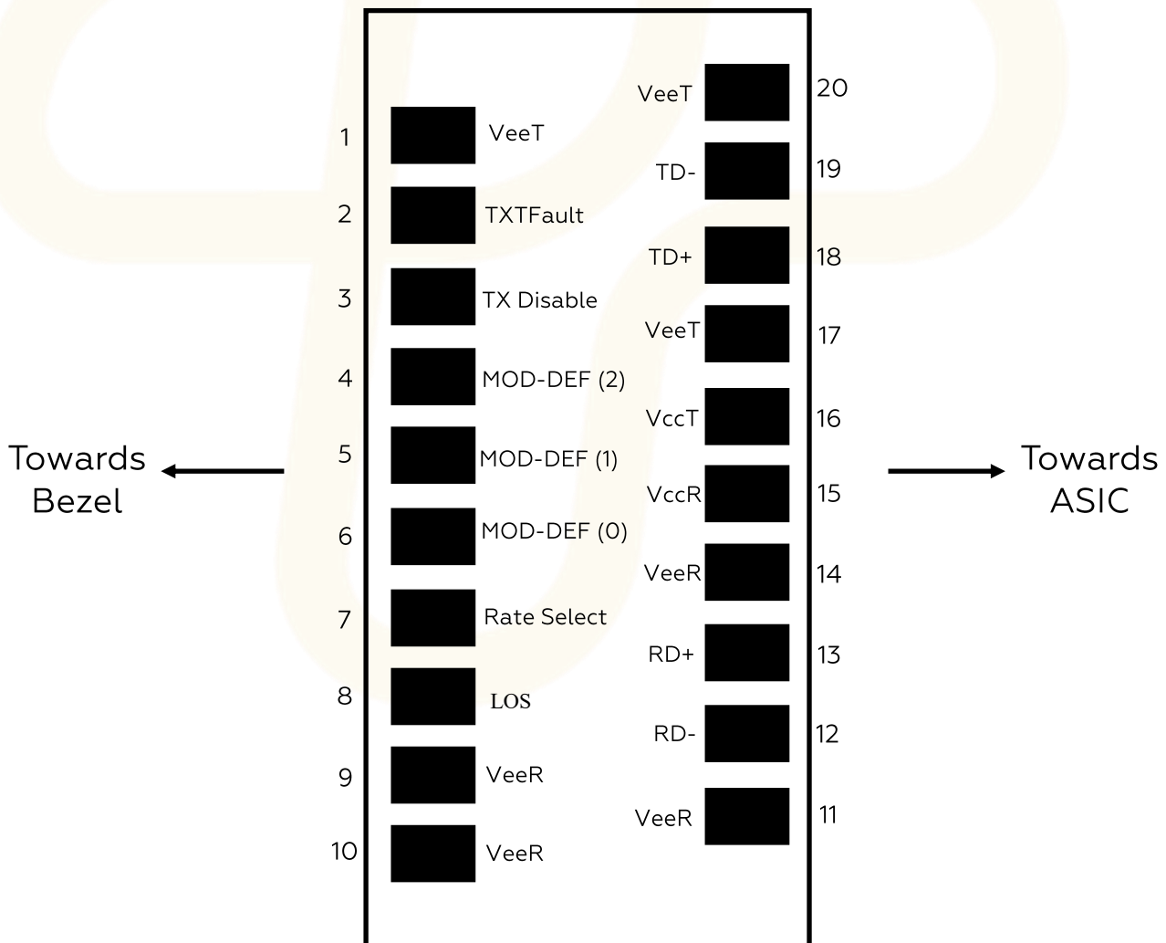
Схема основной платы с выводами
