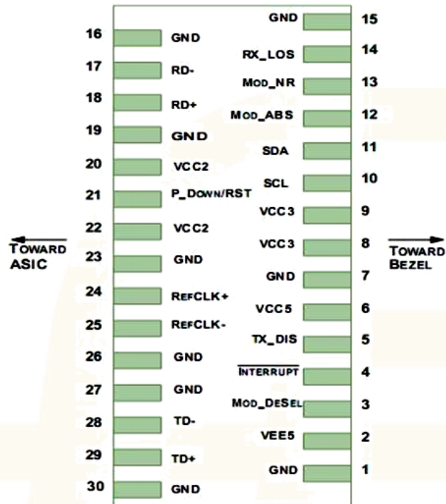
Схема основной платы с выводами
